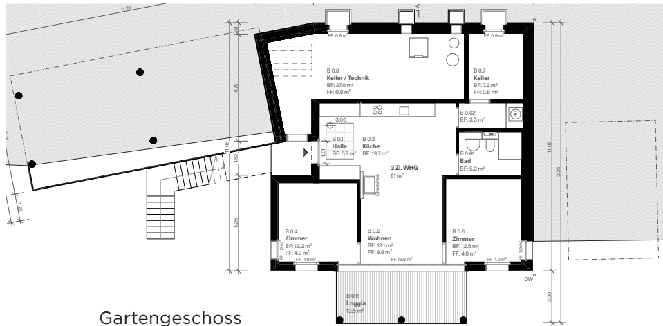
Gartengeschoss
